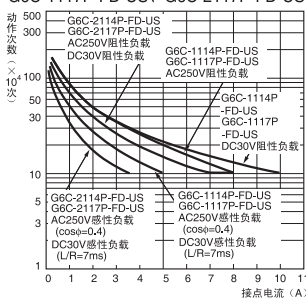
寿命曲线 G6C-1114P-FD-US、G6C-2114P-FD-US G6C-1117P-FD-US、G6C-2117P-FD-US
