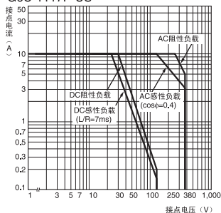
开关容量的最大值 G6C-1114P-FD-US G6C-1117P-FD-US
