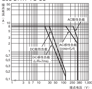
开关容量的最大值 G6C-2114P-FD-US G6C-2117P-FD-US
