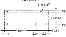
印刷基板加工尺寸 (底视图)
