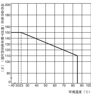
环境温度和最大容许电压
